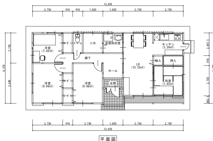
地域振興住宅 4LDK 平面図
