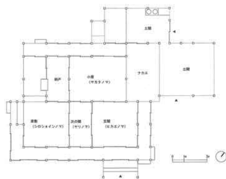
主屋 復元平面図
